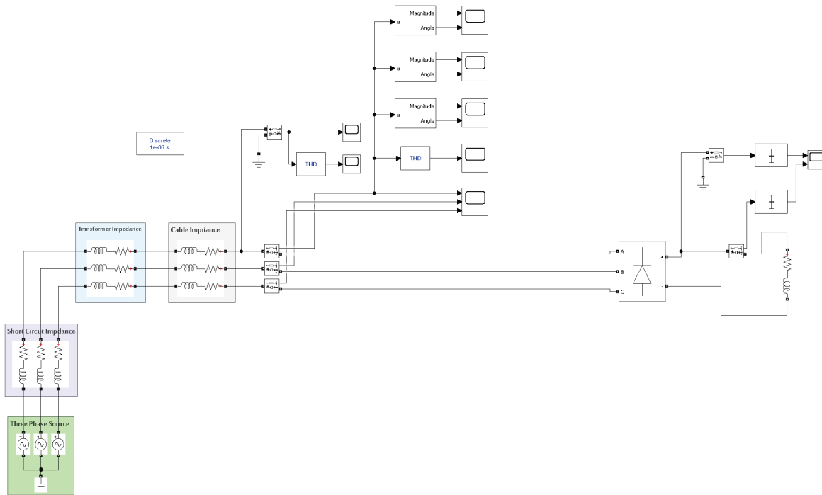
شكل 3: المخطط الكامل للدارة بدون مرشحات
